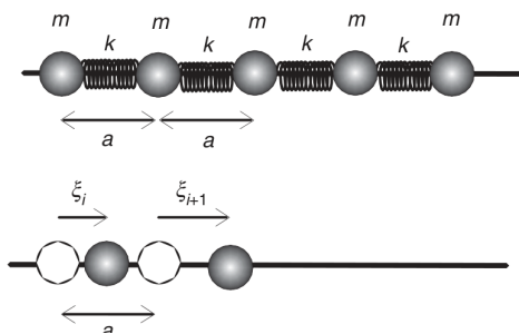
图 8.2: 图 7.2 质量为 m 的珠子穿在一根细而硬的金属丝上, 由劲度系数为 k 的弹簧相连。平衡间距为 a 。下图显示了两颗珠子偏离平衡的距离分别为 \xi_i 和 \xi_{i+1} 。
